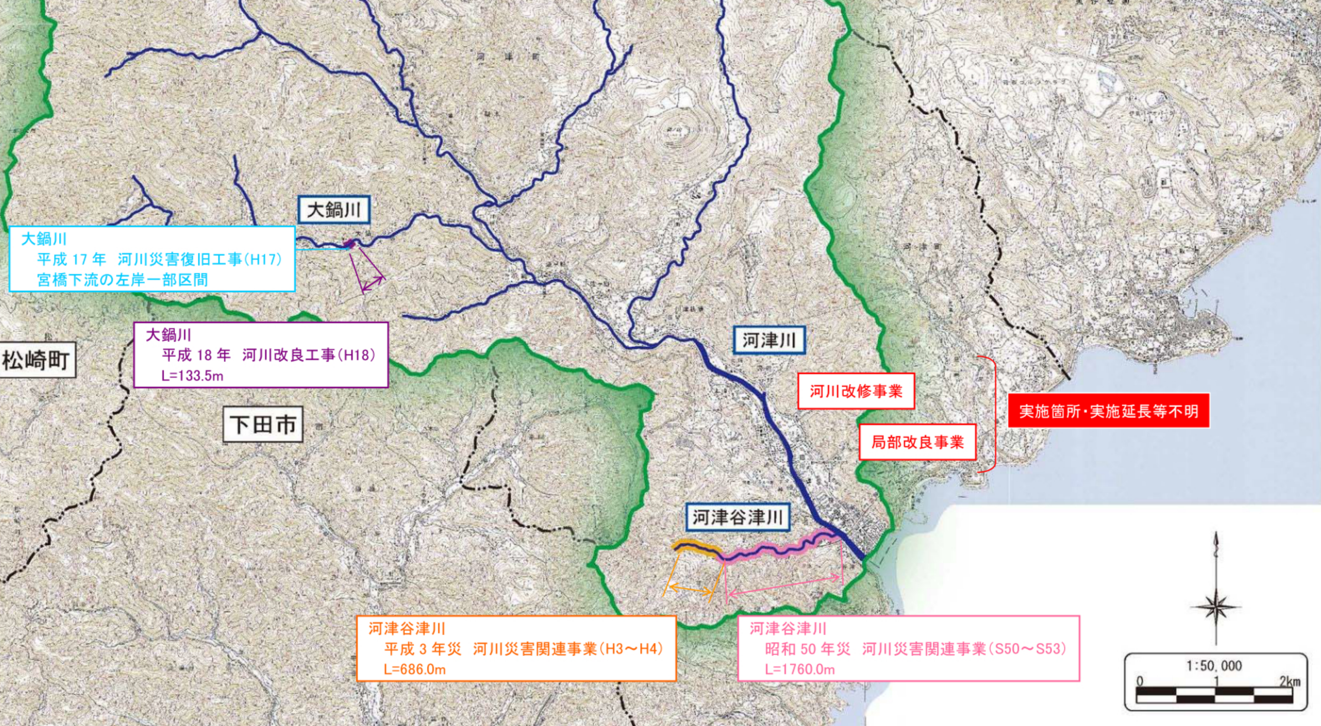
図 5.3.1 治水事業の沿革
